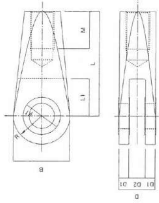
フォークエンド
